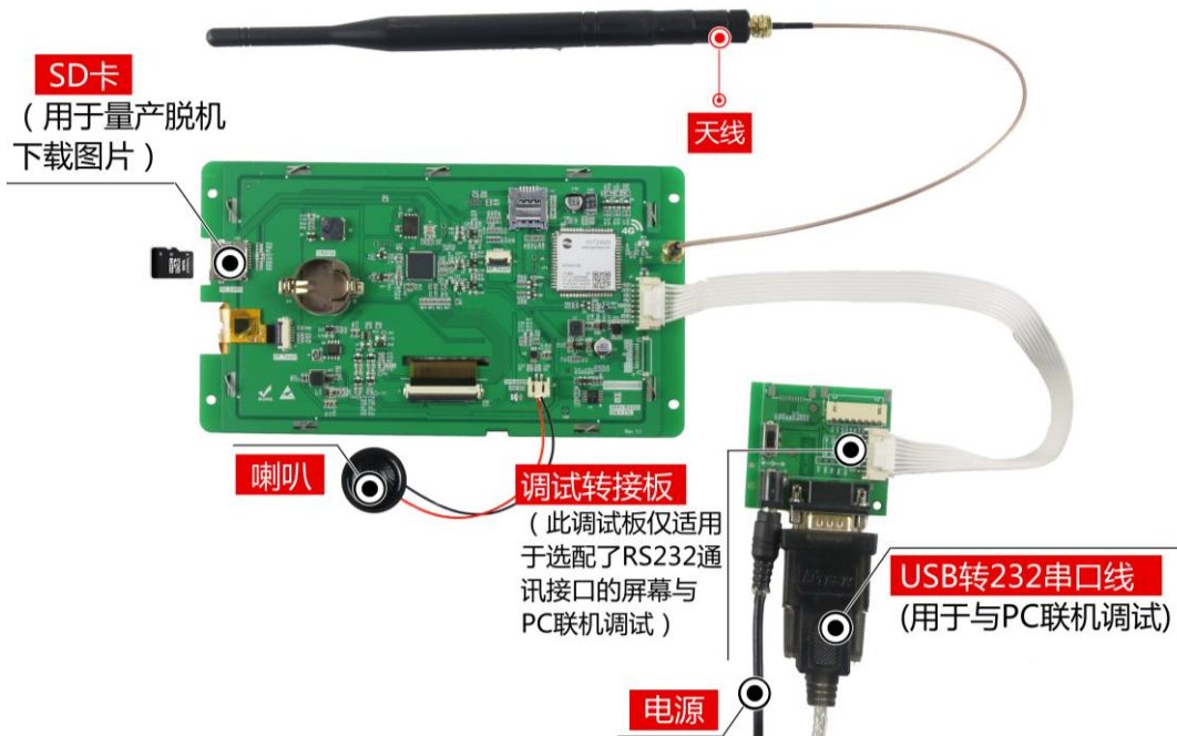
图 1-5 调试工具图
